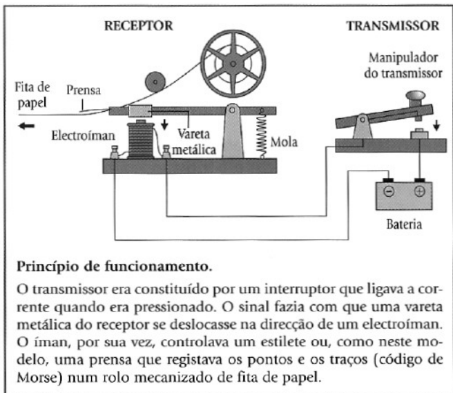
Figura 7 | O telégrafo.
